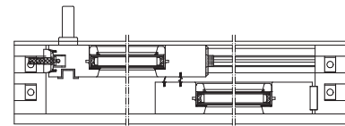
Coupe horizontale
